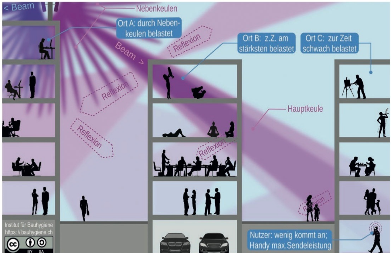
Beam (Strahlenkeule) einer mMIMO-Antenne. Es sind pro Antenne zeitgleich bis zu 8 Beams möglich, die innert Millisekunden laufend ihre Richtung ändern. Auf dem Weg zum Ziel wird der Beam z. T. absorbiert, er durchdringt z. T. Bauteile und wird z. T. an diesen reflektiert/gestreut. Dabei werden Orte unterschiedlich belastet, direkt und indirekt (Reflexion). In der Praxis ist die Strahlungsausbreitung viel komplexer und die Exposition viel heterogener, als in dieser vereinfachten Grafik darstellbar. Nicht zuletzt deshalb sind Messungen und Simulationen mit grossen Unsicherheiten behaftet.
